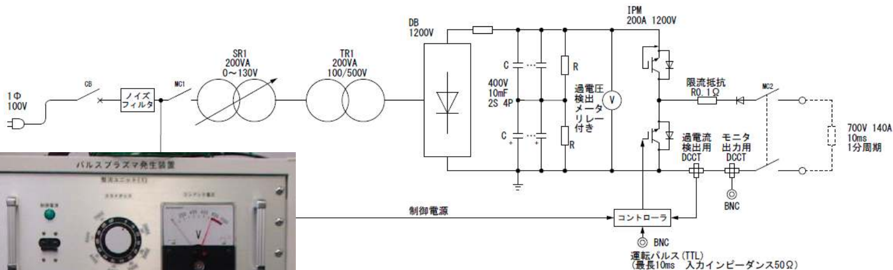
パルスプラズマ発生装置 単線接続図
