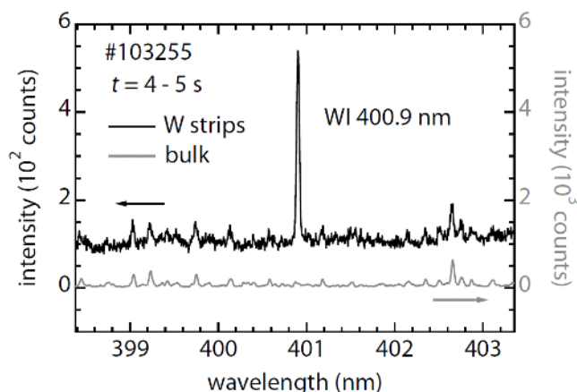
タングステンロッド周辺部とバルクプラズマ中でのWI(400.9nm)スペクトルの比較(#103255)
